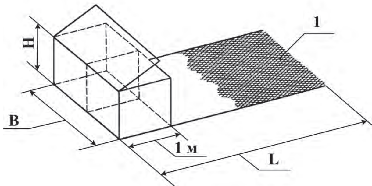
B – ширина короба и армирующей панели; L – длина армирующей панели; H – высота короба; 1 – армирующая панель
