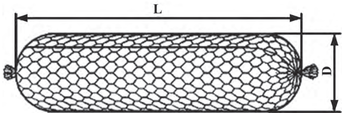
L – длина цилиндрического ГСИ; D – диаметр цилиндрического ГСИ Рисунок А.4 – Конструктивная схема цилиндрических ГСИ
