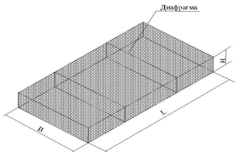
Рисунок.1. Размеры ГСИ.
