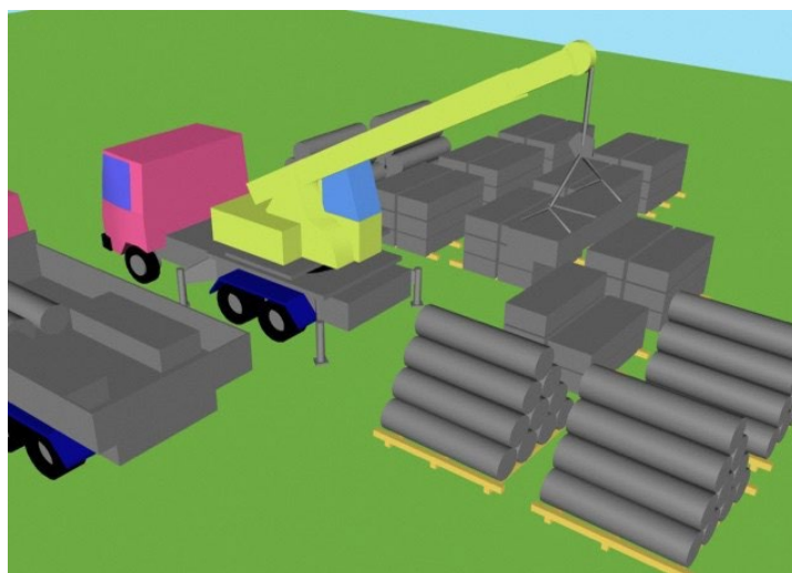
Рисунок.1. Организация склада
