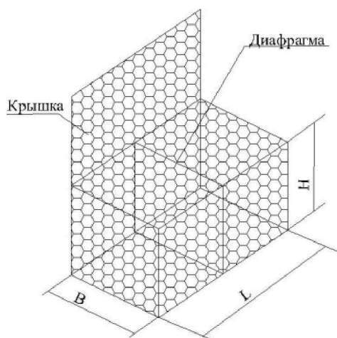
Рисунок 1 — Размеры ГСИ
