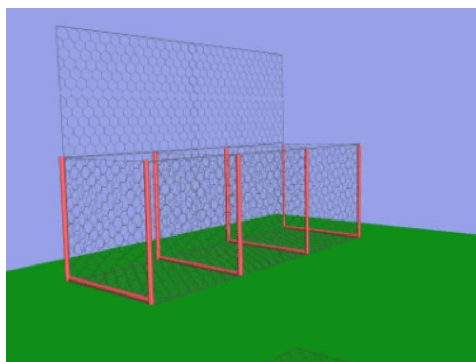
Рисунок 5.4.2 — Собранное коробчатое ГСИ
