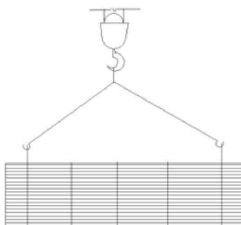
Рисунок 1 — Схема строповки пачки ГСИ
