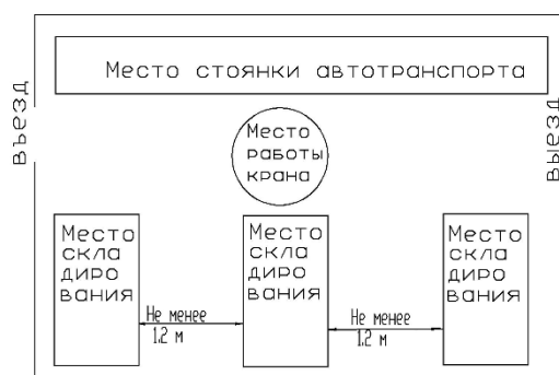
Рисунок 2 — Схема склада
