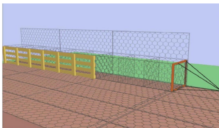
Рисунок 5.4.5 — Вытягивание собранных ГСИ
