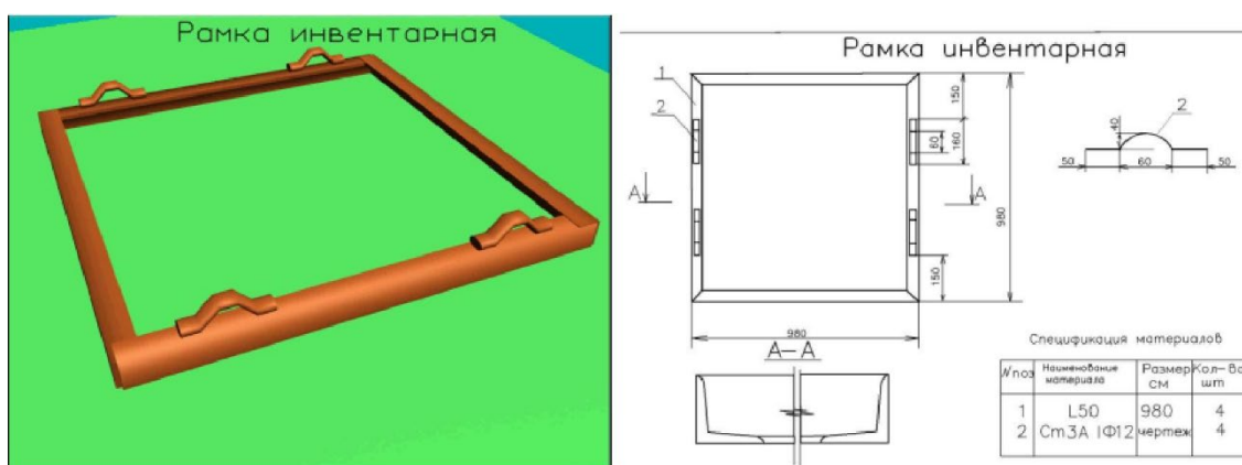
Рисунок 5.4.4 — Рамка инвентарная
