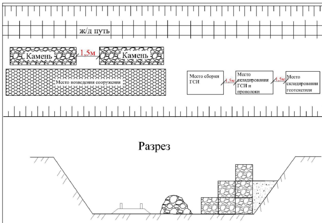
Рисунок 5.3.2 — Организация рабочей зоны при укреплении откосов выемки под ж/д дорогу
