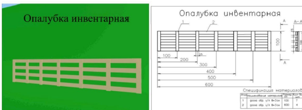
Рисунок 5.4.6 — Опалубка инвентарная
