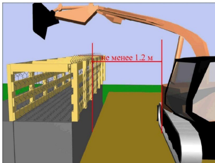
Рисунок 5.А3.4 — Стоянка экскаватора снизу, у лицевой части сооружения
