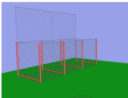
Рисунок 5.А.4.2 — Собранное коробчатое ГСП
