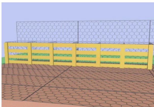
Рисунок 5.4.7 — Установка инвентарной опалубки
