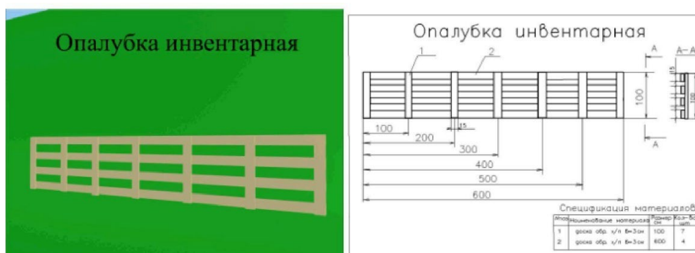
Рисунок 5.А.4.6 — Опалубка инвентарная
