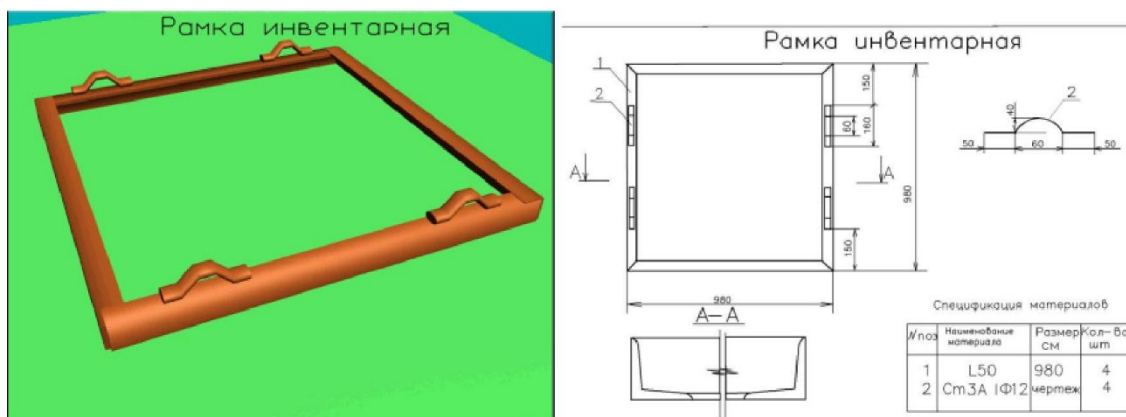
Рисунок 5.А.4.4 — Рамка инвентарная
