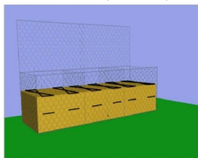
б) заполнение 2/3 высоты ГСИ
