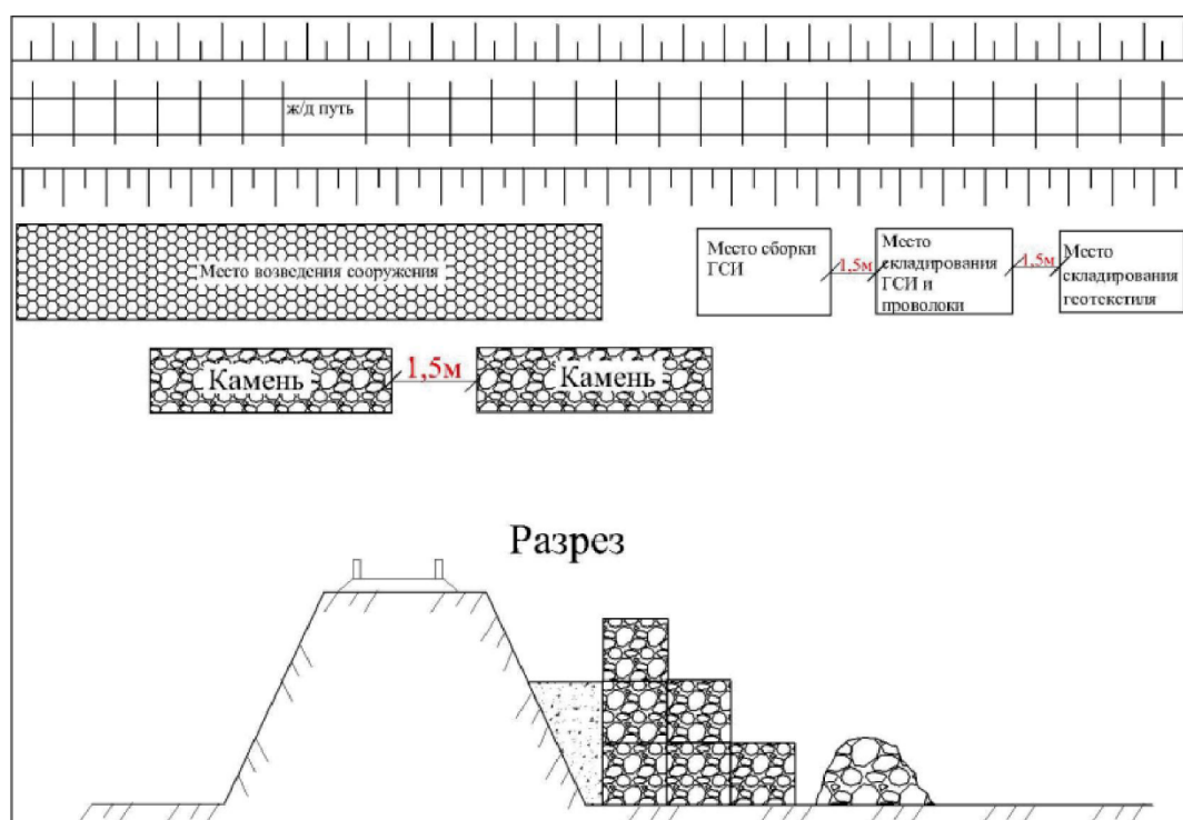
Рисунок 5.А.3.2 — Организация рабочей зоны при укреплении откосов выемки под ж/д дорогу
