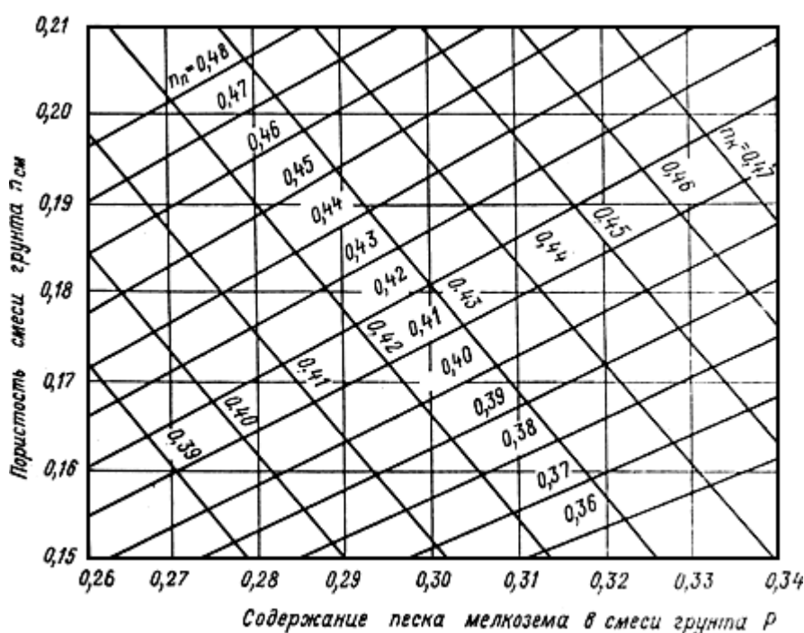
Рис. 5.2. Номограмма для определения физических характеристик смеси грунтов n_{\text{см}} = f(P)
