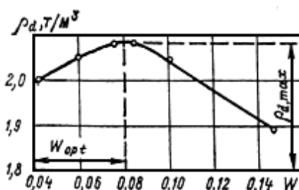
Рис. 20. График зависимости плотности сухого грунта от влажности при виброударном
