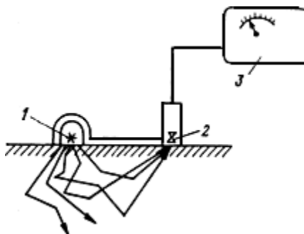
Рис. 45. Поверхностная схема измерений
