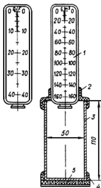
Рис. 31. Трубка СПЕЦГЕО
