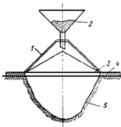
Рис. 2.1. Схема отбора проб грунта методом лунки
