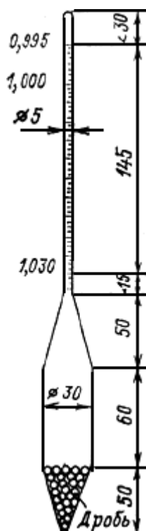
Рис. 6. Ареометр со шкалой 0,995-1,030 и ценой деления 0,001
