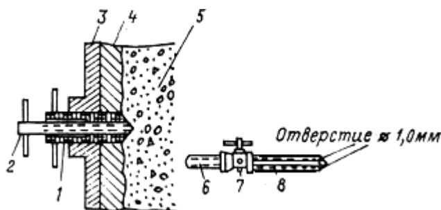
Рис. 54. Конструкция пьезометрического оголовка
