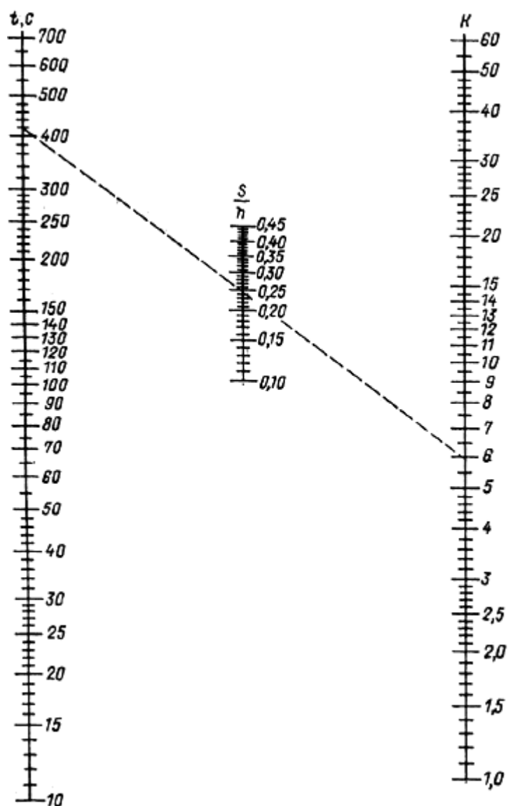
Рис. 30. Номограмма Биндемана для определения коэффициента фильтрации в приборе Каменского
