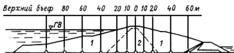
Рис. 4. Пример разбивки створов для отбора проб грунта на поперечнике плотины 1 - боковые зоны; 2 - ядро.
