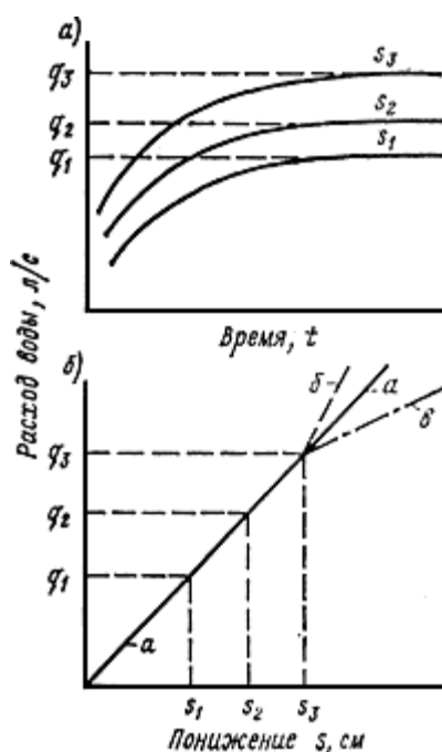
Рис. 48. Зависимость расхода воды q от понижения ее уровня в основании S и времени откачки t (а) и в скважине (б)
