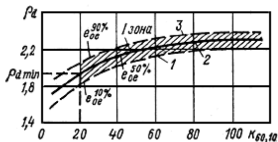
Рис. 60. График зависимости плотности сухого грунта от коэффициента разноразмерности при постоянном значении коэффициента пористости 1 - нижняя граница; 2 - средняя линия; 3 - верхняя граница.
