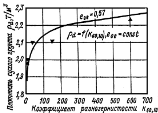
Рис. 64. График зависимости плотности сухих грунтов, уложенных в призмы, переходные
