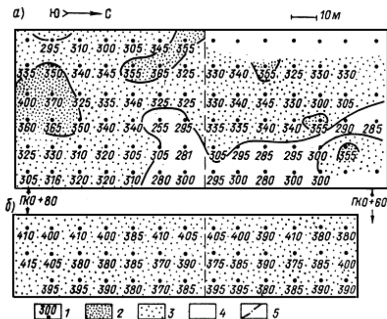
Рис. 42. Поля скоростей v_r в супеях Дангаринской насыпи при ее высоте 16 м.
