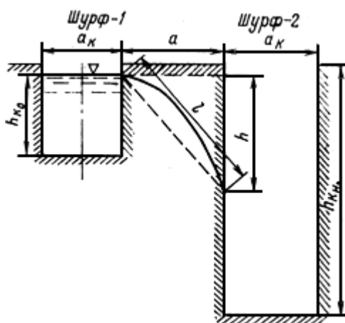
Рис. 51. Схема определения коэффициента фильтрации грунта в полевых условиях методом Семенова
