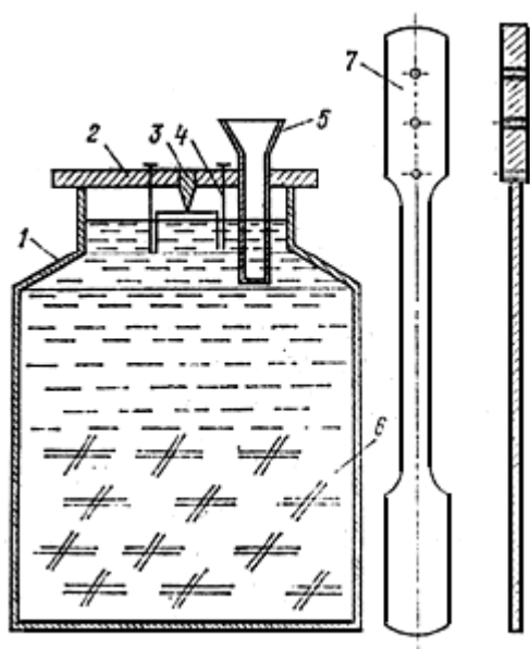
Рис. 8. Прибор для определения влажности грунта объеметрическим методом
