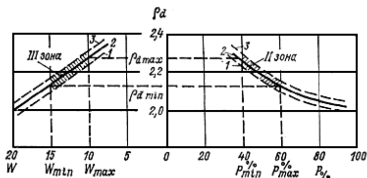
Рис. 63. График зависимости плотности сухого грунта от его влажности и содержания мелкозема в грунте 1 - нижняя граница; 2 - средняя линия; 3 - верхняя граница.
