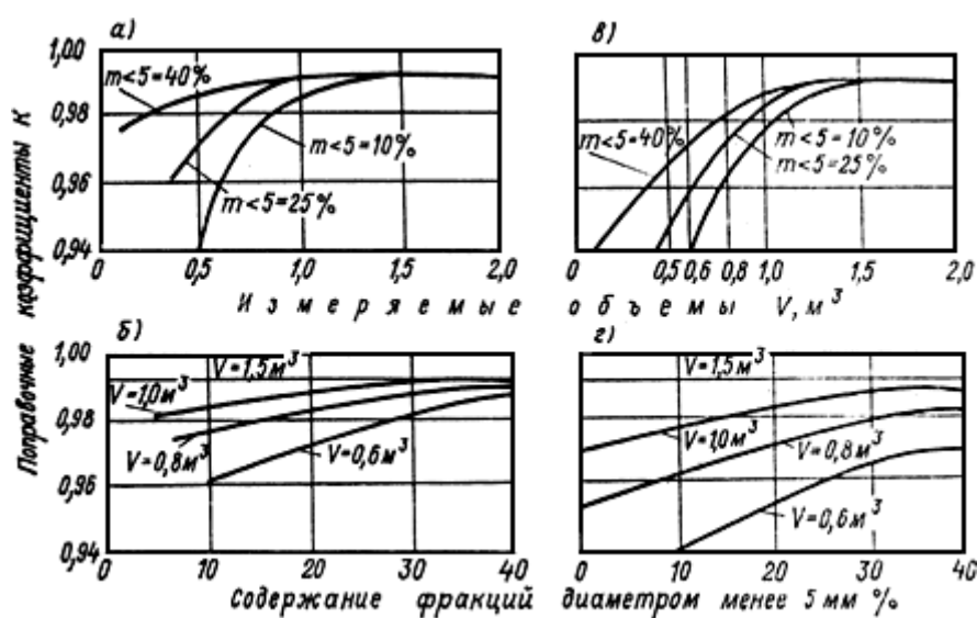
Рис. 2.4. Зависимости поправочных коэффициентов K от измеряемых объемов и содержания в галечнике мелкозема (фракция менее 5 мм)
