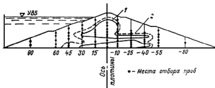
Рис. 70. Изолинии гранулометрического состава намывтого грунта в поперечном сечении плотины
