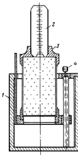
Рис. 33. Прибор КФ-ОМ
