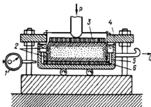
Рис. 24. Срезной прибор для определения прочности песчаных и глинистых грунтов 1 - индикатор часового типа с ценой деления 0,01 мм; 2 - обойма для образца грунта; 3 - штамп; 4 - неподвижная верхняя часть срезной коробки; 5 - подвижная нижняя часть срезной коробки - каретка; 6 - металлическая пластинка с отверстиями.
