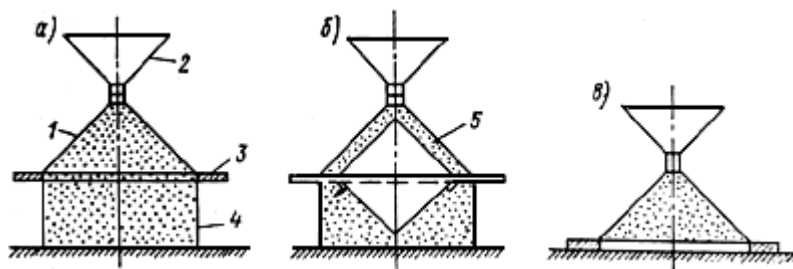
Рис. 2.3. Схема тарировки устройства для определения плотности грунта методом лунки 1 - полый конус; 2 - загрузочная воронка; 3 - плита; 4 - тарировочный бак; 5 - вкладыш.
