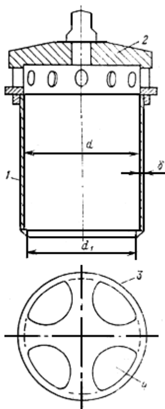
Рис. 5. Пробоотборник
