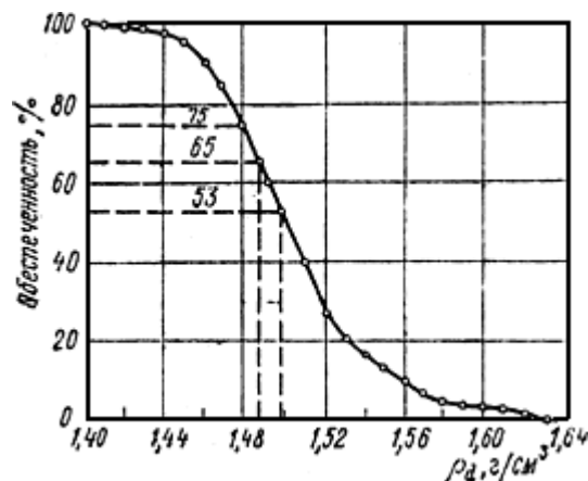
Рис. 67. График обеспеченности плотности сухого грунта
