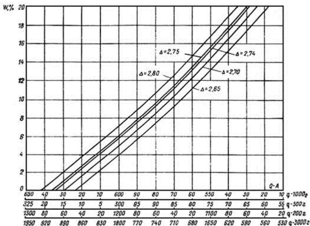
Рис. 9. График для определения влажности грунта объеметрическим методом
