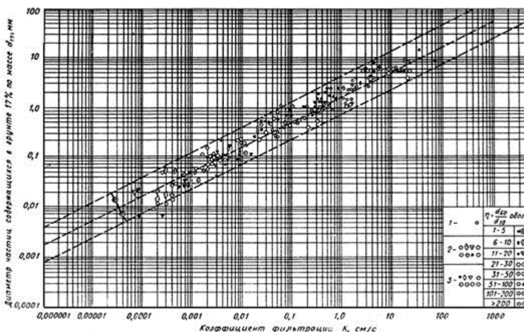
Рис. 56. Экспериментальная зависимость коэффициента фильтрации от величины d_{17} область рыхлой смеси грунта: K_{60,10} > 1 ; область плотной смеси грунта: K_{60,10} > 1 ; 1 - коэффициент фильтрации щебенистого грунта, полученный в лабораторных условиях; 2 - грунты, коэффициент фильтрации которых получен в натурных условиях; 3 - грунты, коэффициент фильтрации которых получен в лабораторных условиях.
