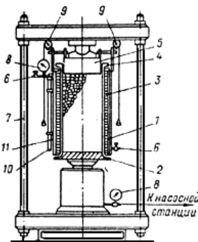
Рис. 27. Схема прибора СШ-240
