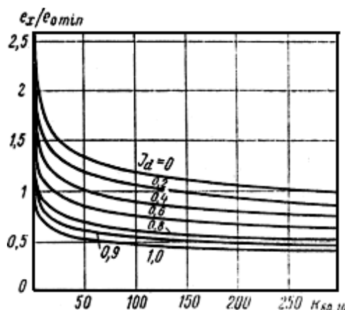
Рис. 4.2. График зависимости относительных приведенных значений пористости от коэффициента разнотерности
