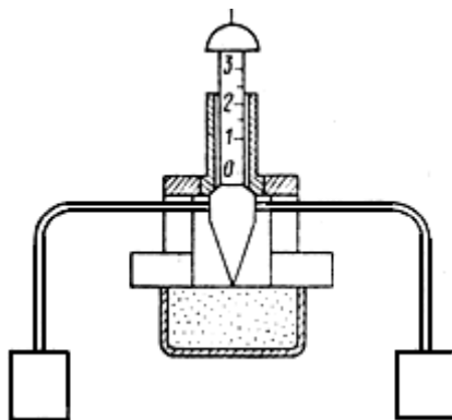
Рис. 11. Усовершенствованный балансирный конус, ППГ
