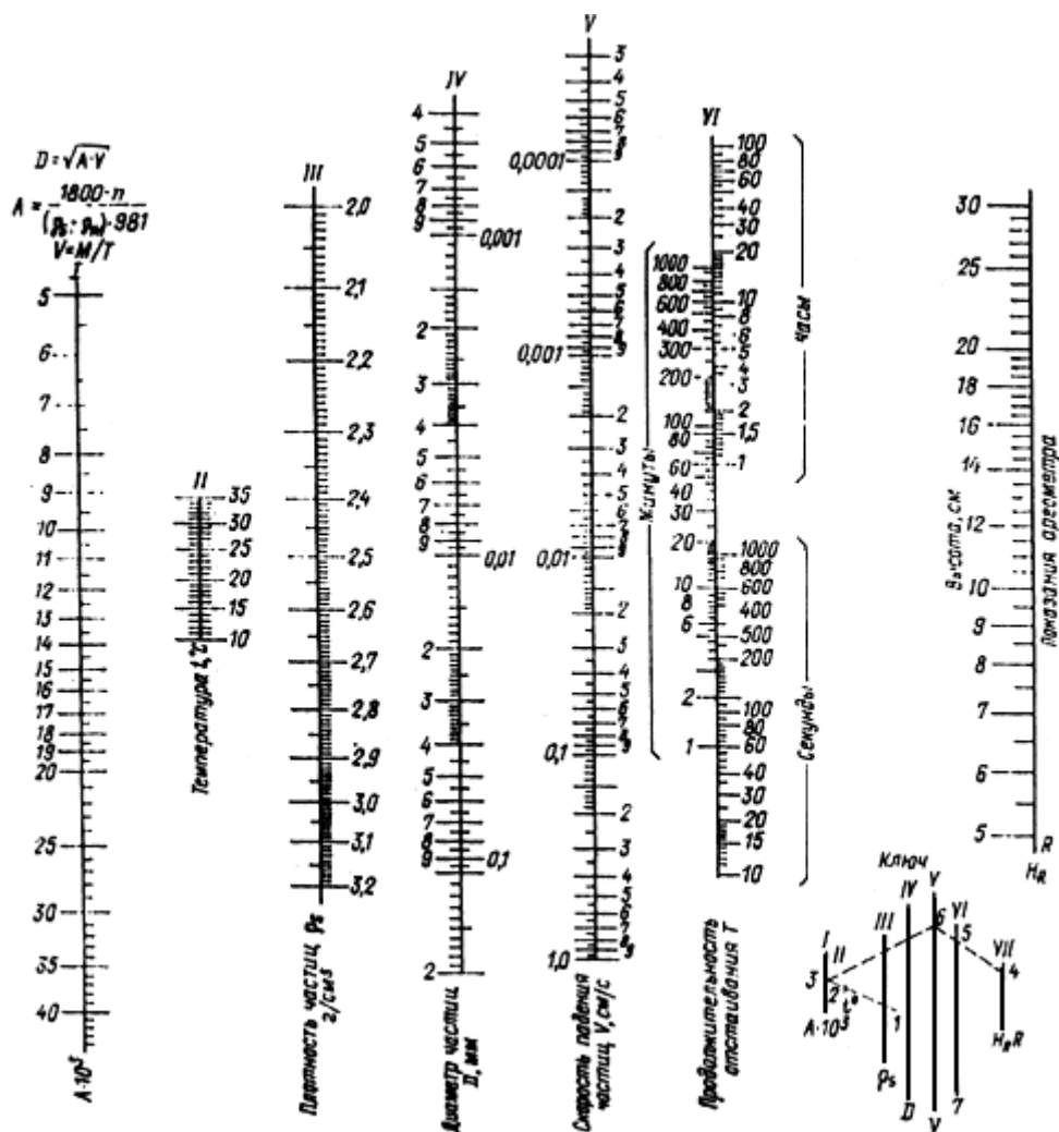
Рис. 7. Номограмма для ареометрического анализа. Арабские цифры в ключе - порядок хода определений
