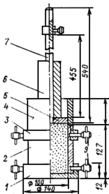
Рис. 12. Схема прибора СоюздорНИИ для стандартного уплотнения грунтов 1 - поддон; 2 - разъемный цилиндр емкостью 1000 см 3 ; 3 - кольцо; 4 - насадка; 5 - наковальня; 6 - груз массой 2,5 кг; 7 - направляющий стержень; 8 - ограничительное кольцо; 9 - зажимные винты.
