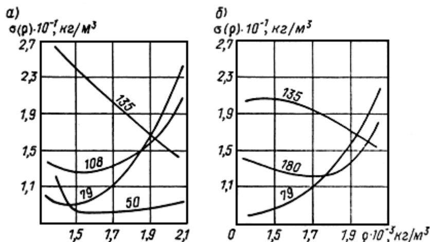
Рис. 3.3. Зависимость средней квадратической абсолютной погрешности измерения плотности s(r) от ее абсолютных значений для сухих (а) и водозаполненных (б) скважин различного диаметра
