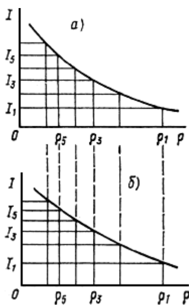
Рис. 3.2. Пример градуировки радиоизотопных влагоплотномеров при помощи эквивалентов влажности и плотности. Градуировочный график, полученный на стандартных образцах (а) и на эквивалентах (б) I_i - интенсивность регистрируемого излучения для i -го ( i = 1, 2, 3, \dots ) значения параметра \rho_i .
