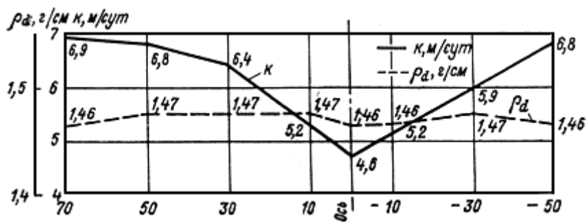
Рис. 68. График изменения плотности сухого намытого грунта и коэффициента фильтрации в пределах яруса сооружения (для неоднородной плотины)
