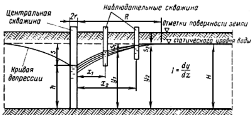
Рис. 47. Расчетная схема определения коэффициента фильтрации в полевых условиях методом откачки
