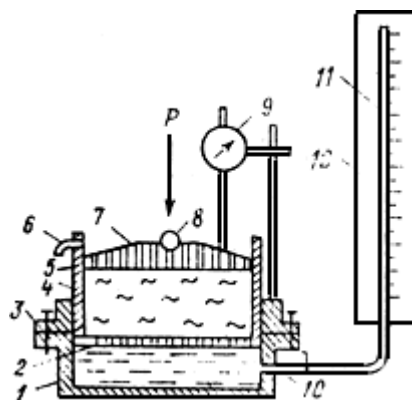
Рис. 34. Принципиальная схема конструкции компрессионно-фильтрационного прибора
