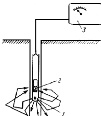
Рис. 46. Глубинная схема измерений
