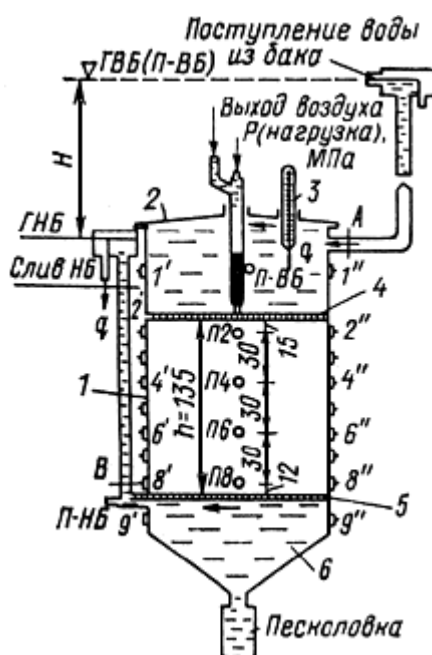
Рис. 36. Схема вертикального фильтрационного прибора ВНИИГ
