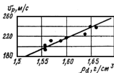
Рис. 40. Зависимость скорости v_p от плотности сухого грунта для намывных песков (слой 1 м) по данным Е.В. Чебасовой
