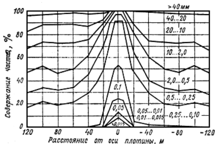
Рис. 66. График фракционирования намывного грунта
