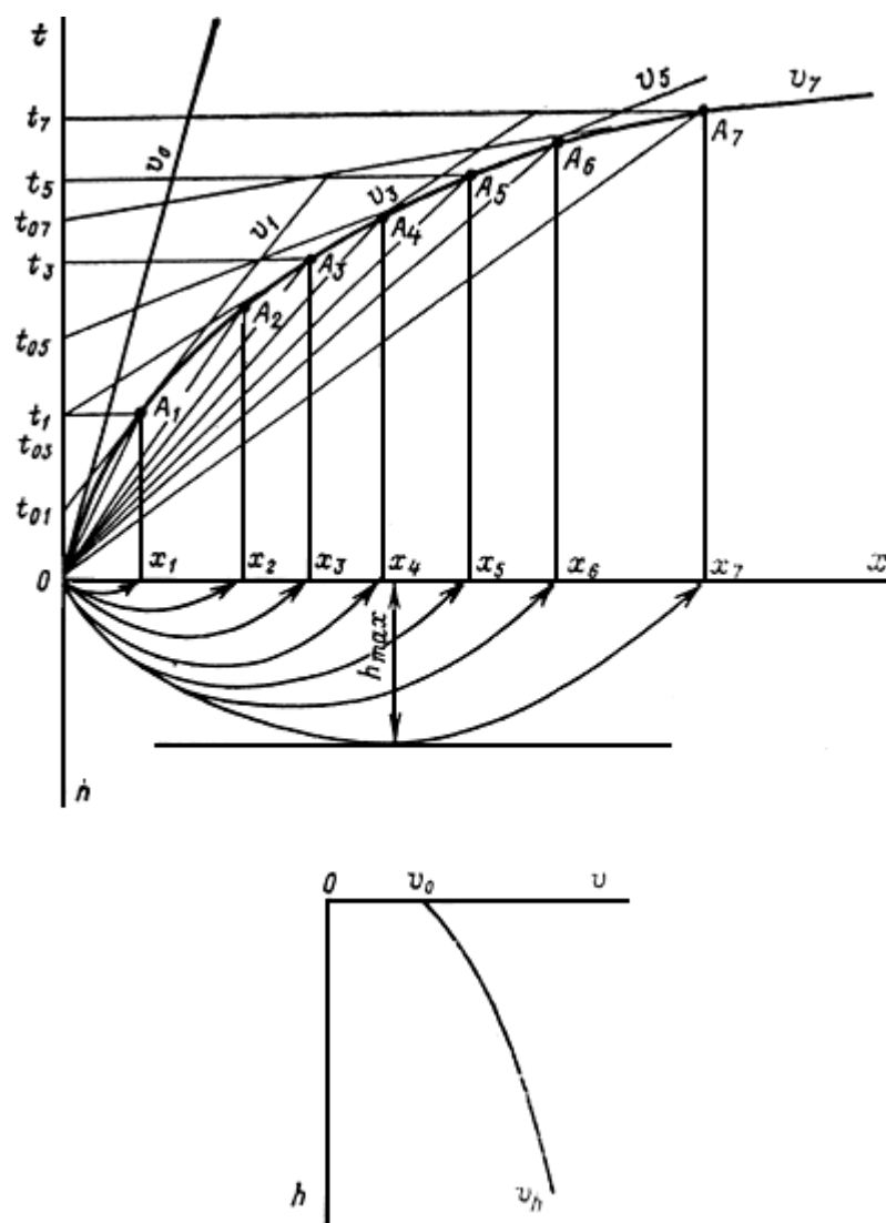
Рис. 43. Годограф рефрагированных волн, схема хода лучей упругих волн в градиентной среде и график изменения скорости по глубине
