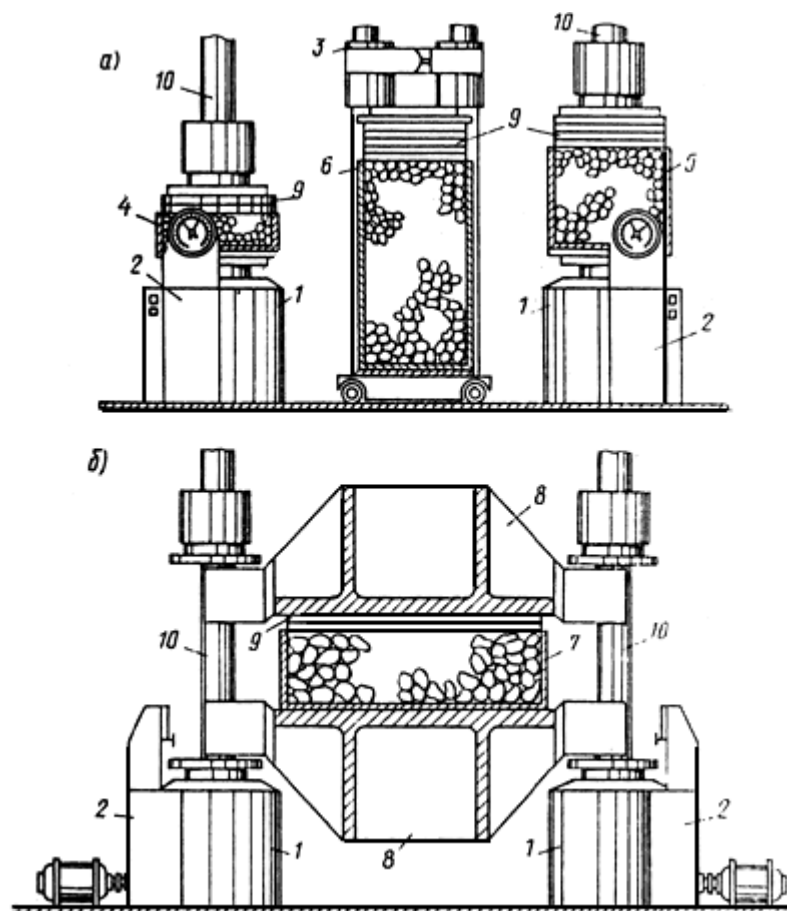
Рис. 23. Компрессионные приборы
