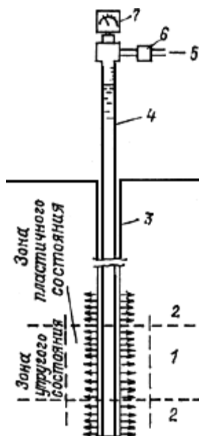
Рис. 57. Схема прессиометра (по Луи Менару)
